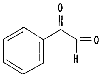
PHENYLGLYOXAL
